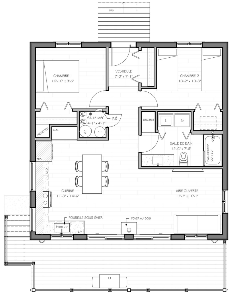
PLAN AMÉNAGEMENT REZ-DE-JARDIN
